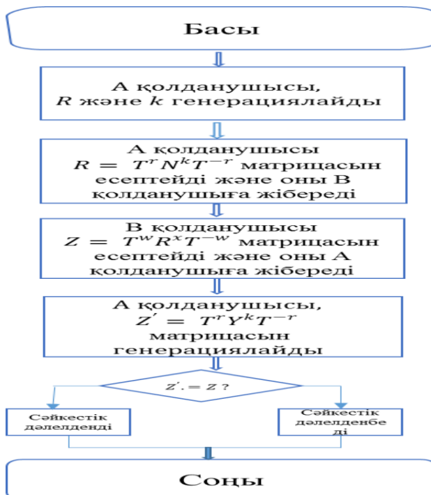
2- Сурет. Кері матрицаға негізделген нөлдік жариялаумен сәйкестендіру әдісі
