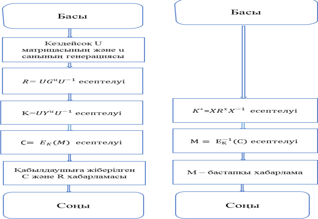
1- Сурет. Кері матрицаға негізделген ашық түрдегі шифрлау және шифрды ашу
